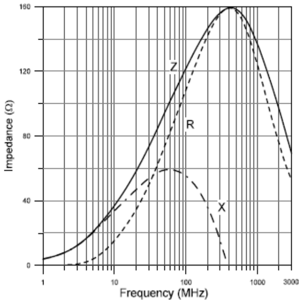
CB 4532-121
