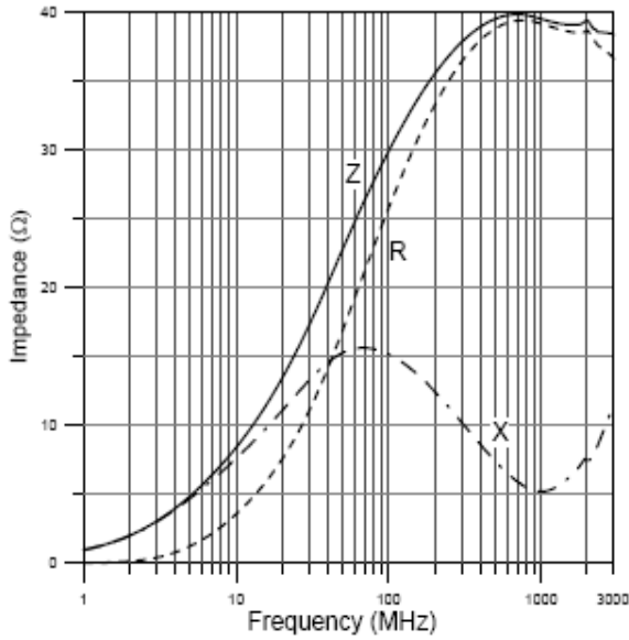
CB 4532-310
