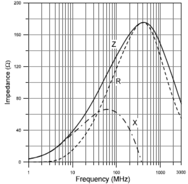
CB 4532-151
