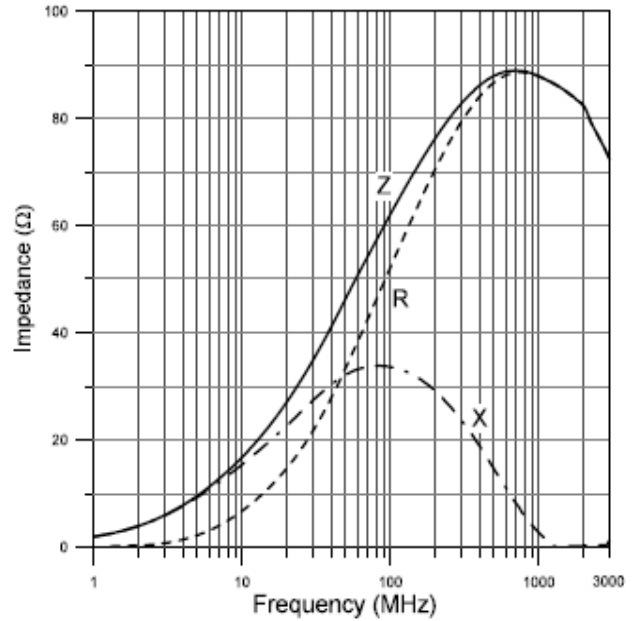
CB 4532-600
